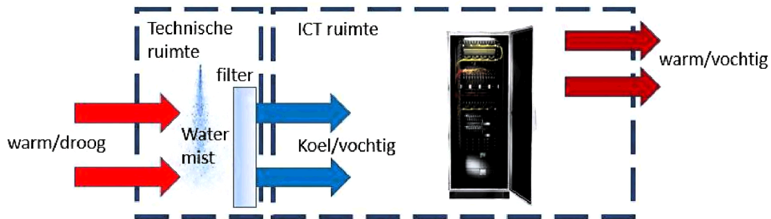
Figuur 5 Schematische voorstelling van directe luchtkoeling met verdamping [20] (■■■■■, 2023)
