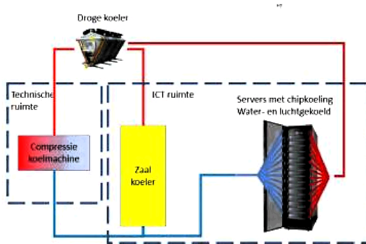
Figuur 8 Schematische voorstelling van direct-op-chip koeling [20] (■■■■■, 2023)
