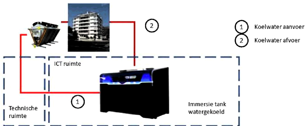
Figuur 9 Schematische voorstelling immersie koeling met directe verbinding met een warmtenet [20] (■■■■■, 2023)
